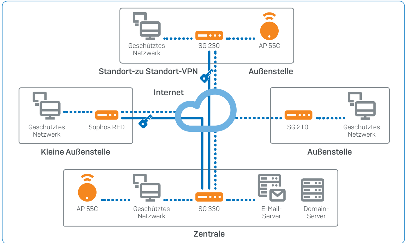
Szenario mit SG Series Appliances und RED für Außenstellen
